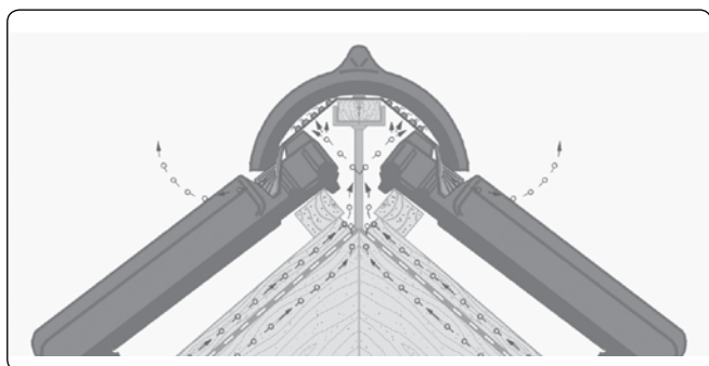
Standard nock, med nocktätningrulle
