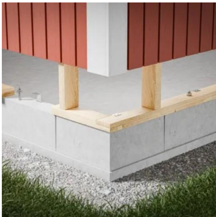
The base element G-sockeln.
