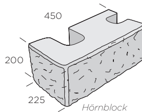
Hörnblock
