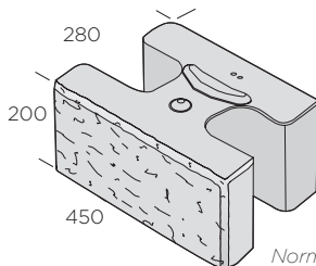
Normalblock
