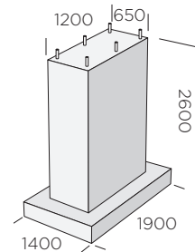
Sugtransformatorfundament
