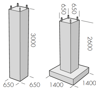
Kontaktledningsfundament
