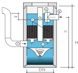
Funktionskiss TMA
