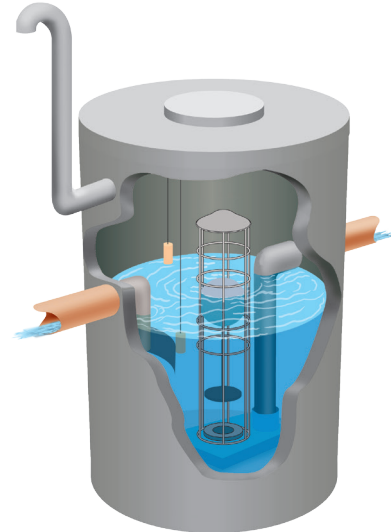
Oljeavskiljare OA 3-50 (med särskild utrustning)
