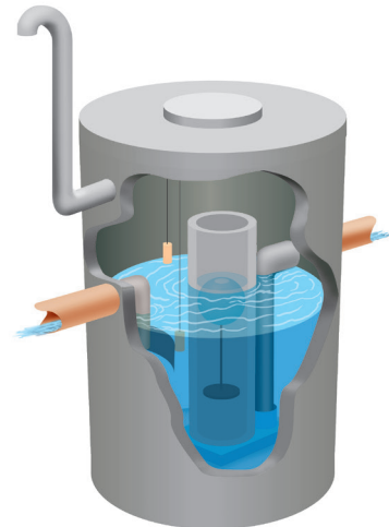
Koalescensavskiljare KA (med särskild utrustning)
