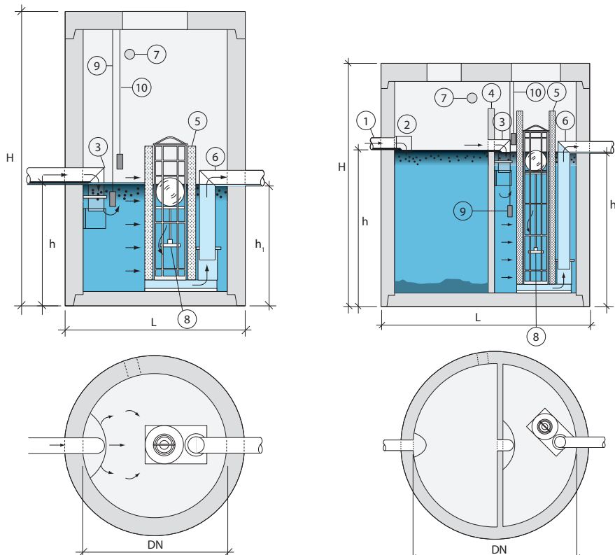
Koalescensavskiljare KA (med särskild utrustning)
