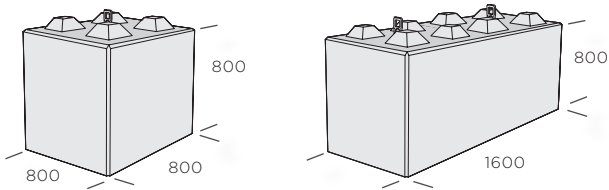
Flexiblock levereras med ingjutna kulankare, se avsnitt hjälpmedel.
