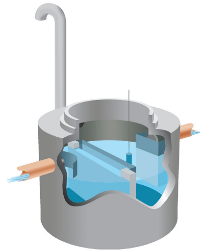
Fettavskiljare FA (med särskild utrustning)
