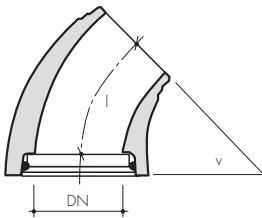
1. Krokrör, Oarmerade rör - KANMAX PG®)
