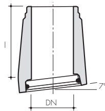
2. Vinkelrör (Oarmerade rör - KANMAX PG®)
