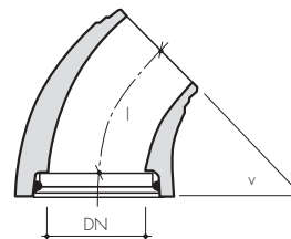
3. Krokrör (Armerade rör - GERMAX®)
