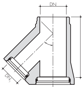
Grenrör 45° (Oarmerade rör - KANMAX PG)
