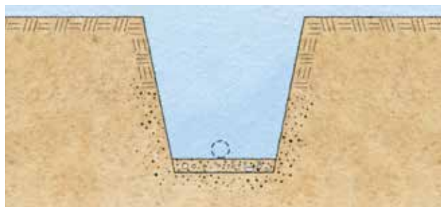
Grundläggning siltjord
