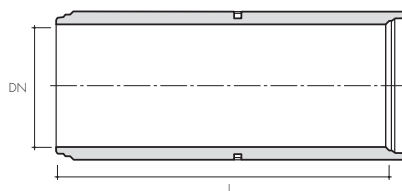
2. Rakt rör (Armerade rör - GERMAX*)
