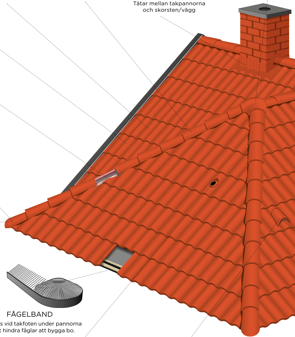
TVÅKUPIG TAKPANNA
